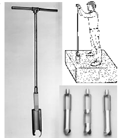
0230-200 筒式土钻 (图中由左到右) 0232D2-100 沙土土钻筒 0231D2-100 泥浆土钻筒 0230D2-100 土钻筒
